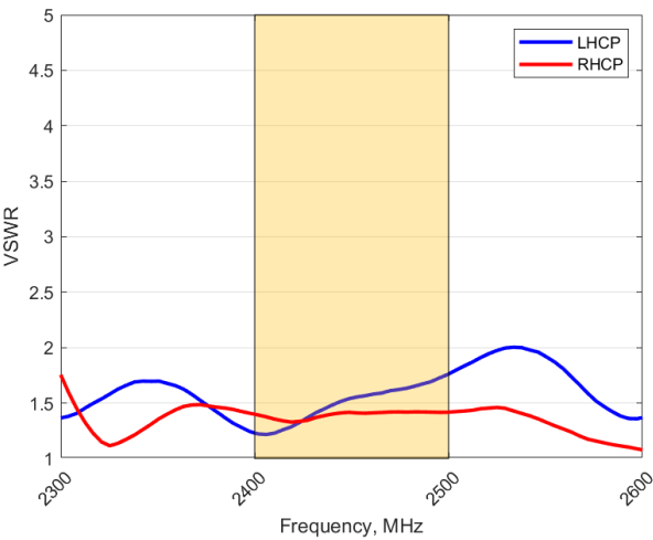
VSWR: 2400 – 2500 MHz
