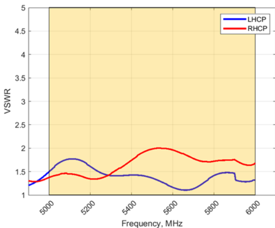
VSWR: 5000 – 6000 MHz
