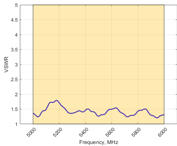
VSWR
